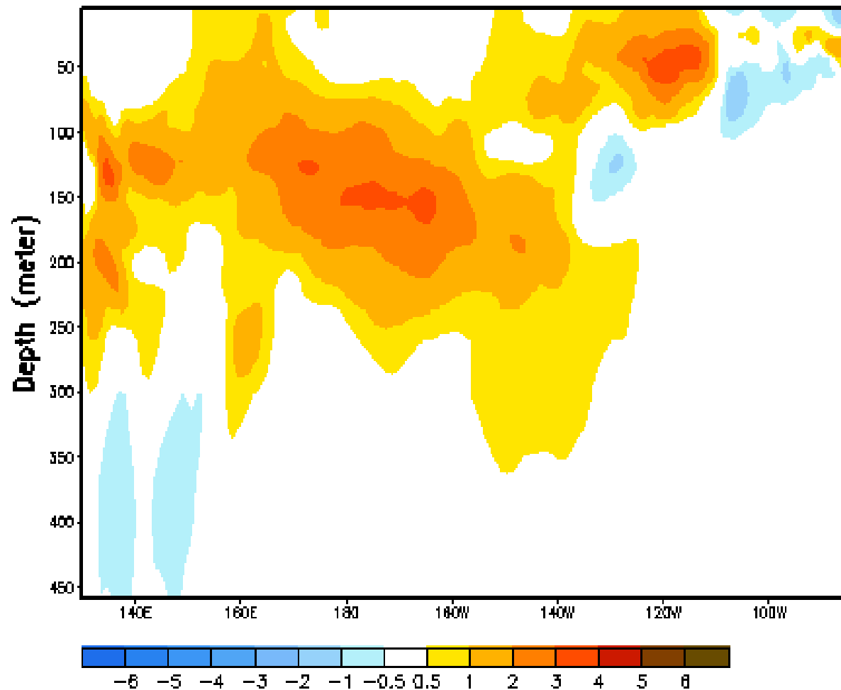
Equatorial Temperature Anomaly (°C)
